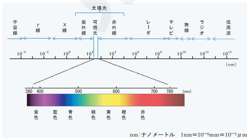
図3 電磁波・光の波長と色
